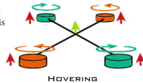
HOVERING
